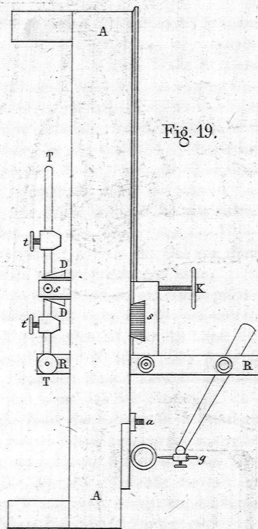
Colladon's Gasreinigungssapparat.
