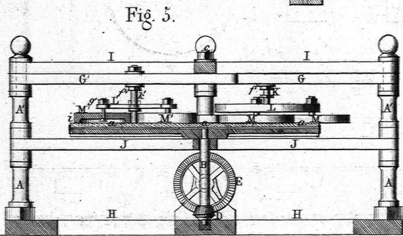
Lindsay's Maschine zum Poliren v. Glas, Marmor etc.
