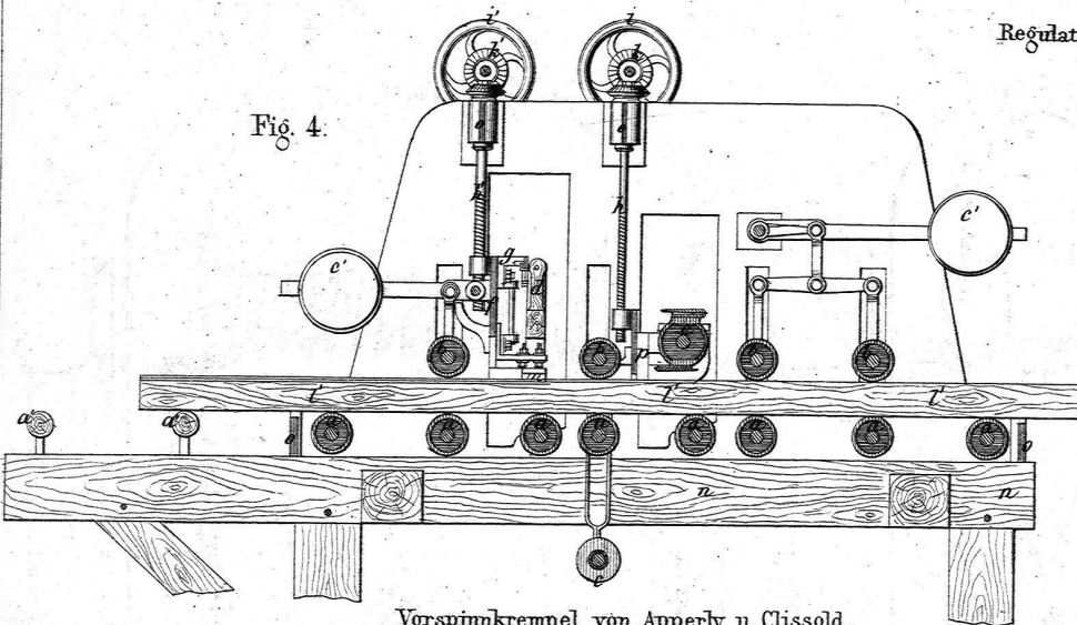
Vorspinnkrempe von Apperly u. Clissold.
