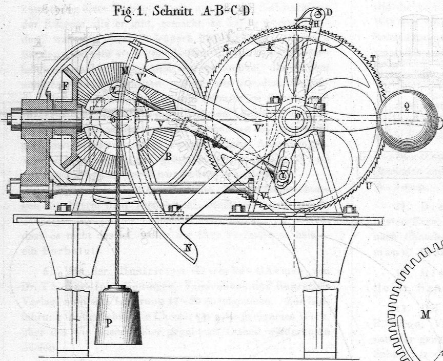
Totalisirende Dynamometer von Moison, Noury u. Matter.
