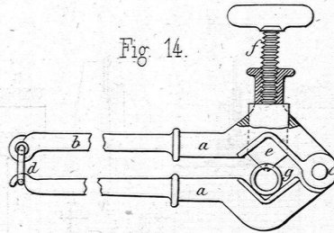
Werkzeug zum Zerschneiden von Metallröhren..
