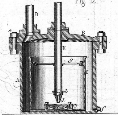
Wassersfang bei Dampfkesseln. Fig. 12.
