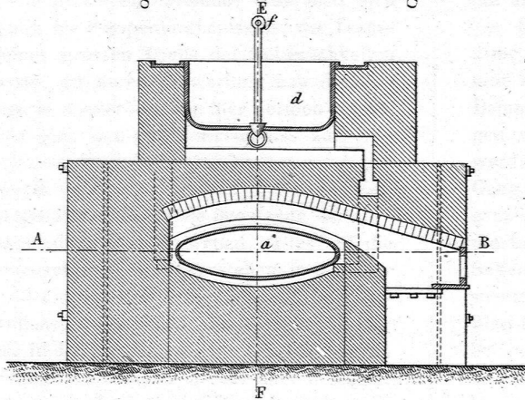
Fig. 3. Grundriss nach A-B der Fig. 2.
