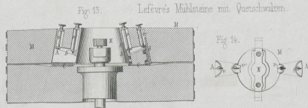
Fig. 13. Lefevre's Muehlsteine mit Quetschwalzen.
