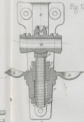
Wandlager leichte Transmissionswellen.
