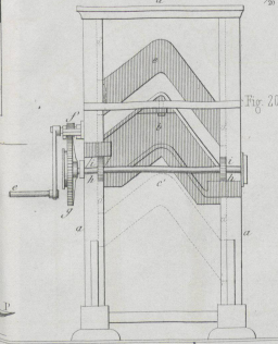
Walkmaschine für Stiefelschäfte.
