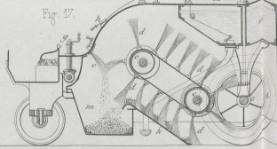
Apparat zum Messen u. Wägen des Getreides.
