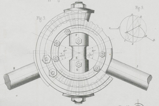
Blees' Universal Kuppelung.
