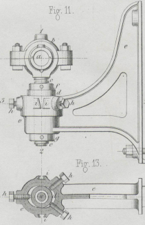
Wandlager leichte Transmissionswellen.
