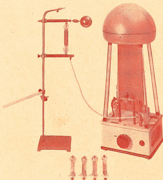
Bandgenerator mit Gegenkugel und Geißleröhren
