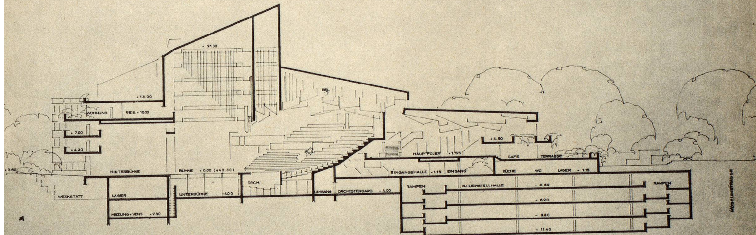
ANGESSCHNITT A - A
