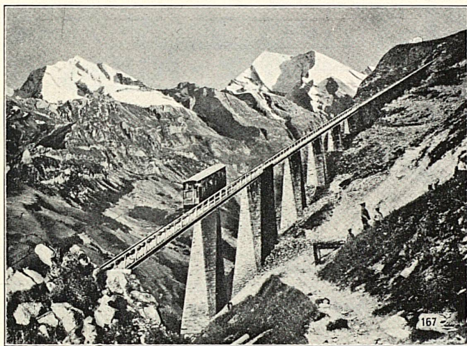
SEILBAHN NIESEN, Berner Oberland. Totale Länge 3496 m, überwindene Höhe 1643 m, Maximalsteigung 68%
