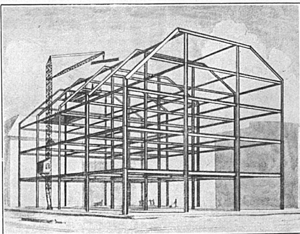
Stahlskelett zum Neubau Industrie- und Handelshaus zum „Graggenthor“ der Firma J. A. Kuhn & Co. Luzern
