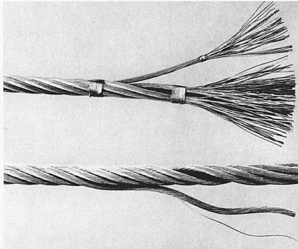
Oben: Drahtseil 15 mm Durchmesser, 222 x 0,7 mm, verzinkter Stahldraht mit 180–200 kg/mm 2 Bruchfestigkeit, nicht vorgeformt
