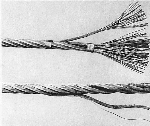
Oben: Drahtseil 15 mm Durchmesser, 222 x 0,7 mm, verzinkter Stahldraht mit 180–200 kg/mm 2 Bruchfestigkeit, nicht vorgeformt
