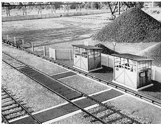
40 T WAGGON-WAAGEN OHNE GELEISEUNTERBECHUNG
