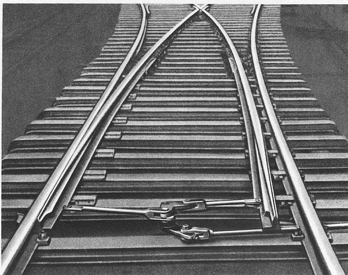
Federzungenweiche mit «Simplex»-Zungenverschluß
