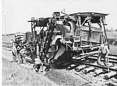
Cribleuse
