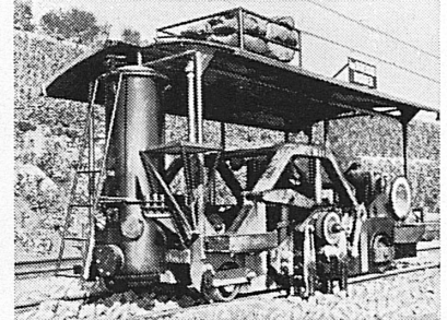
Bourreuse
