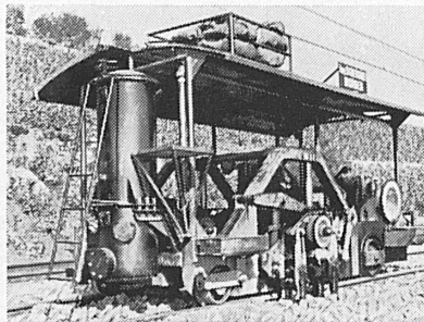
Bourreuse
