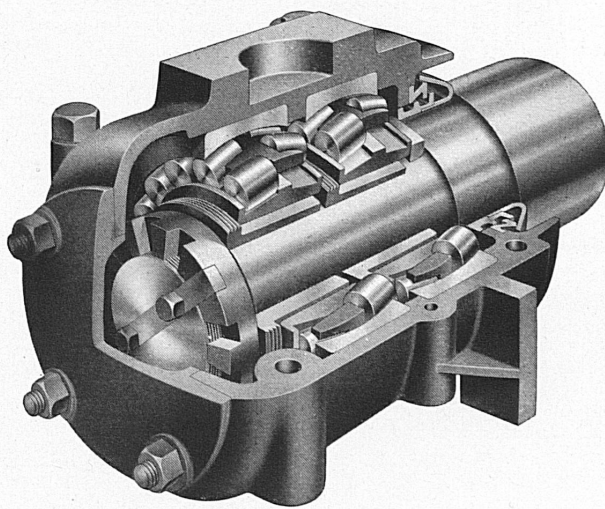
Achsbüchse mit Pendelrollenlagern
