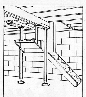
Unten: die Simplex-Stahlspindel-Spießwinde wird direkt in die Holzkolonne eingebaut, um als permanente Spannvorrichtung zu dienen.
