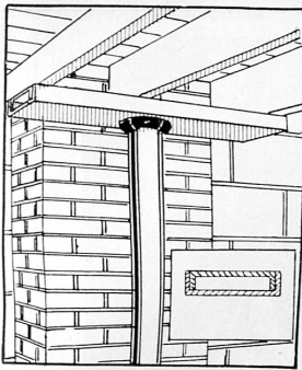
Unten: LMZ-Stahlrohrdeckenstütze (Längsschnitt), mit welcher Röhren verschiedener Ausführung, mit 100 mm Lichtweite, verwendet werden können. Nur einige der mannigfaltigen Anwendungsmöglichkeiten sind oben symbolisch dargestellt.
