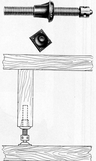
Unten: die Simplex-Stahlspindel-Spießwinde wird direkt in die Holzkolonne eingebaut, um als permanente Spannvorrichtung zu dienen.
