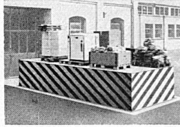
Hydraulische Hebebühne für den rationellen Auf- und Abblad von Fahrzeugen. Hubkraft 6000 kg
