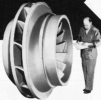
Francisrad «Ferrera», Gewicht 4,6 t +GF+ Stahlguss mit 13% Chrom
