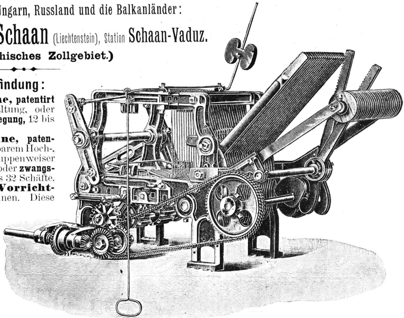
Offenbach-Schaffmaschine, doppelhebend, mit zwangsläufiger Cylinderbewegung. Gros-de-tour-Vorrichtung und Hakenauskehrung.
