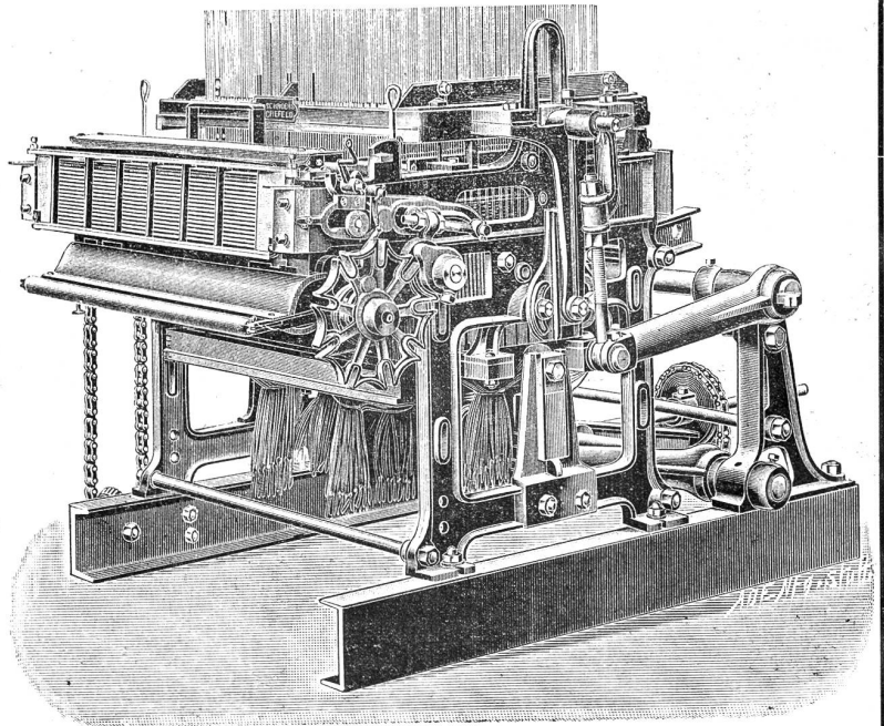
Feinstich-Jacquardmaschine für endlose Papierkarte mit zwangsweiser rotierender Karten-Cylinderbewegung.
