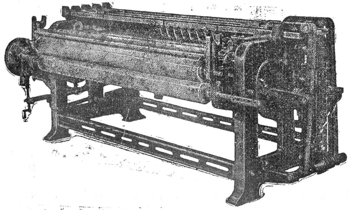
Diese Reibmaschine gegen die Mühle rühmend mit Messerschlitzen. System Simonin. Ceci est une machine à rebroussement avec chariot à laine. Mes. système Simonin.
