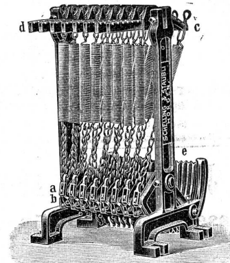
Federzugregister
