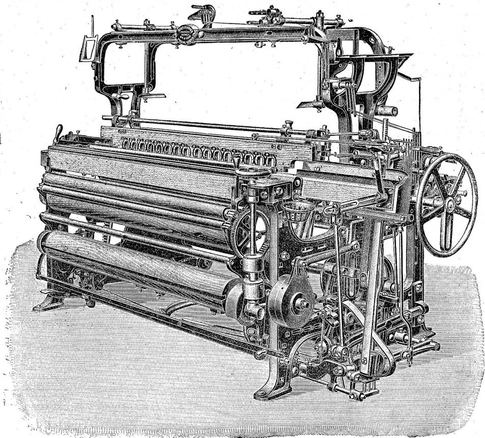
Einschütziger Brochierwebstuhl mit Kreislade.
