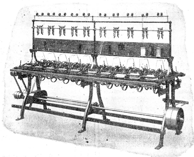
Patent-Kreuzwinde-Maschine eingerichtet zur Herstellung von Größe-Kreuzspulen ab Putz-Spulen.
