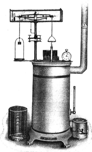
Gangbarste Grösse: Für Versuche bis 500 gr. und mehr. Zur Bestimmung des Feuchtigkeitsgehaltes loser Textil-Rohstoffe und Garne von Wolle, Seide, Baumwolle, (Papier-Rohstoffe, Holzschliff etc.). Für Spiritus-, Gas- oder elektrische Heizung. Neueste solide Ausführung mit feinsten Präzisions- Wage in metallgefasstem Glasgehäuse, Drahtkorb, Hakenkranz, Thermometer, Wasserwage, Gewichtssatz
