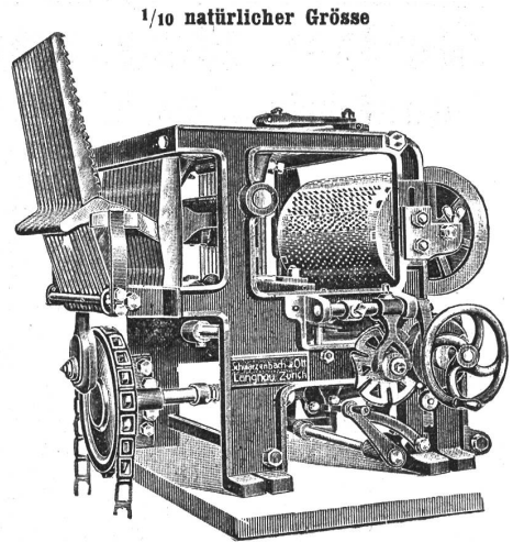
Doppelhub-Schaffmaschine „Reform“
