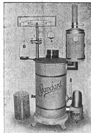
Conditionierapparat zur Bestimmung der in Rohmaterial oder Garnen, Seide, Baumwolle, Wolle etc. enthaltenen Feuchtigkeit.
