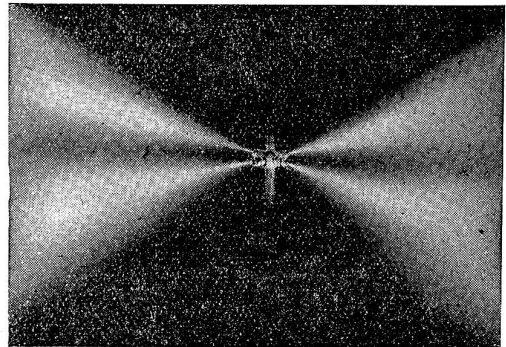
Vierdüsiger Zerstäuber mit Druckluftbetrieb
