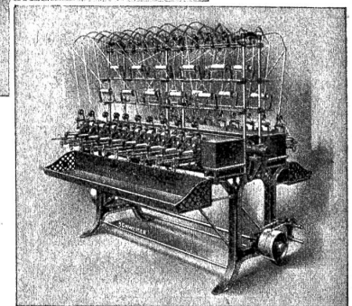
Kreuzschuß-Spulmaschine Typ BUA. „Klein-Rapid“
