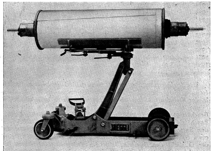
Abb. 5 Hydraulischer Kettbaum-Hubwagen
