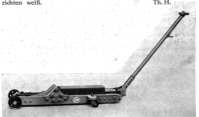
Abb. 6 Hydraulischer Autoheber
