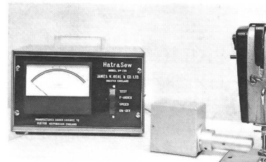
HATRASEW Stickschaden-Prüfgerät
