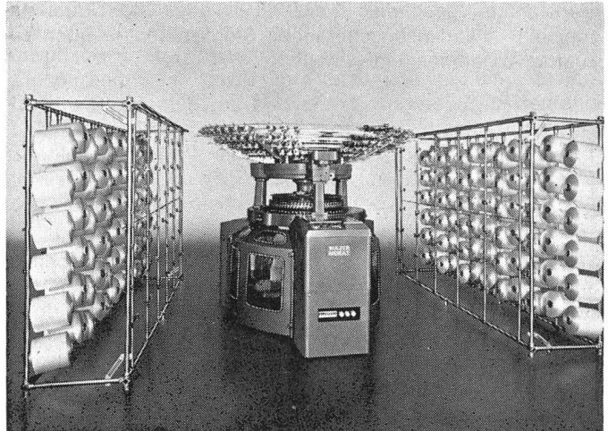
144systemige Interlock-Rundstrickmaschine IL 144 der Firma Sulzer Morat GmbH
