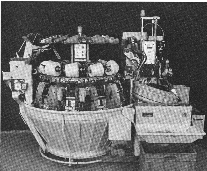
Schweiter-Coner CA 12 D
