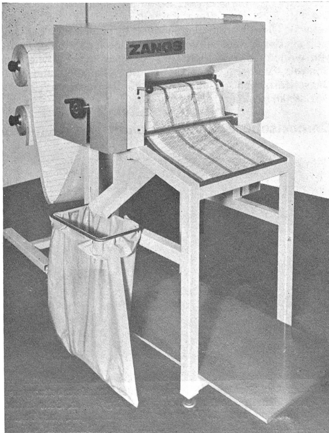
Kartenschnellstanze Patropunch® 528 innerhalb des Zangs-Patrocard-Systems® 525, einem rechnergesteuerten Verarbeitungssystem der Jacquard-Ateliertechnik, mit Abrolleinrichtung 527 für gerolltes Kartenpapier.
