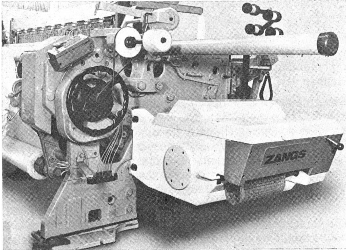
Zangs-Gegenzug-Rotationsschaftmaschine 440 für vielschäftiges Weben bei hohen Touren und grosser Blattbreite.
