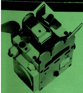
Splicer oder Knoter auf allen Schweiter-Conern leicht auswechselbar
