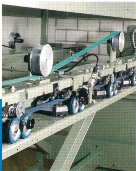
Prüfstand für Tangentialriemen
