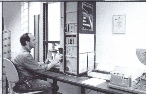
Scheitelstauchwert- Ermittlung
