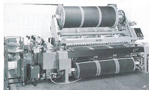
Abb. 10: Picanol-Günne Frotterwebmaschine (Luftdüse)
