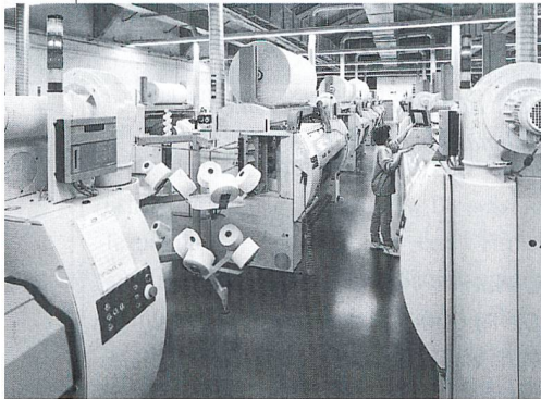
Abb. 1: Die Reibenschwebmaschine M8300 von Sulzer Textil
