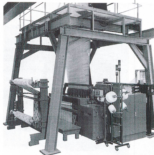
Abb. 11: Picanol-Günne Doppelflor-Greiferwebmaschine
