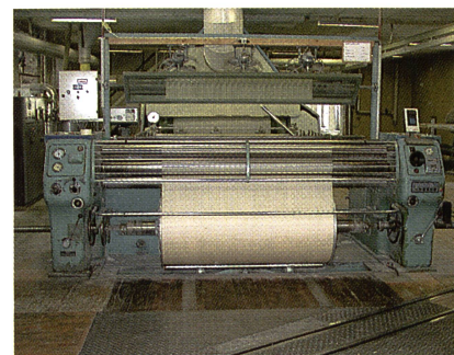
Schlichtmaschine
