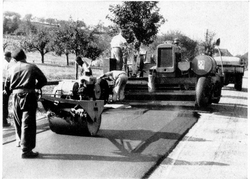
Einbau Teppichbelag Erlen mit Straßenfertiger
