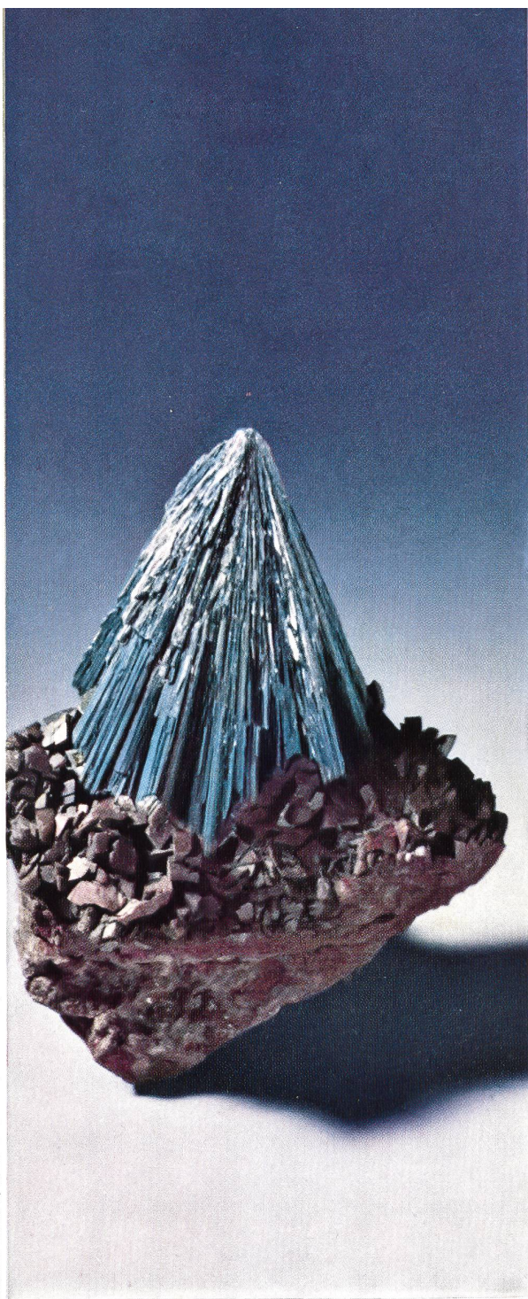
Stibine radiée, avec sidérose, Carinthie, Autriche
