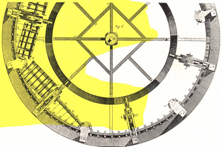
Detail of a twisting loom - XVIII the century engraving - Dictionnaire raisonné des sciences
