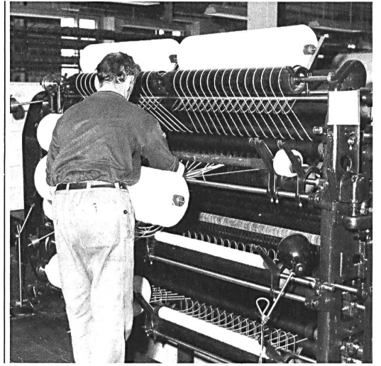
Entnahme der Vorgarne auf dem Streichgarnkrempe. Enlèvement des mèches de préparation de la cardé. Removal of the roving from the carding machine.
