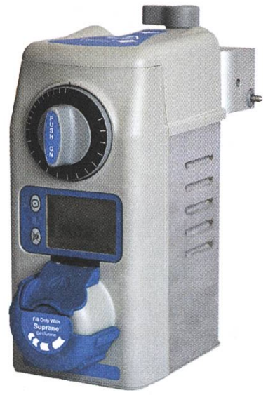
Anästhesieverdampfer für Narkosemittel basierend auf Sensirion-Technologie. (Penlon, UK)
