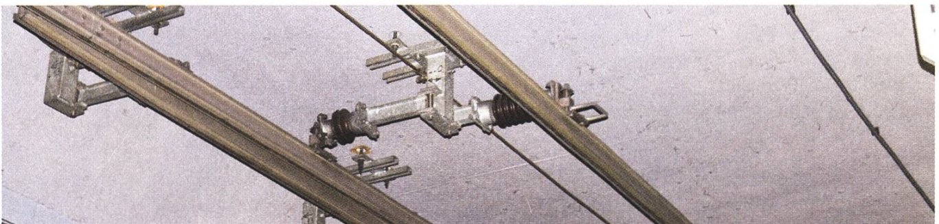
Doppelte Fahrleitung für die Sihltal- und Uetlibergbahn
