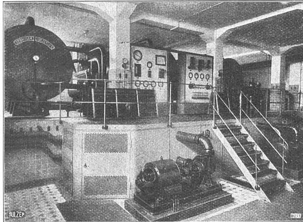
Fernheizung in der Heilanstalt Eglfing. Heizzentrale mit Wärmespeichern, Umwälzpumpen, Fernthermometeranlage und zentraler Regulierstation
