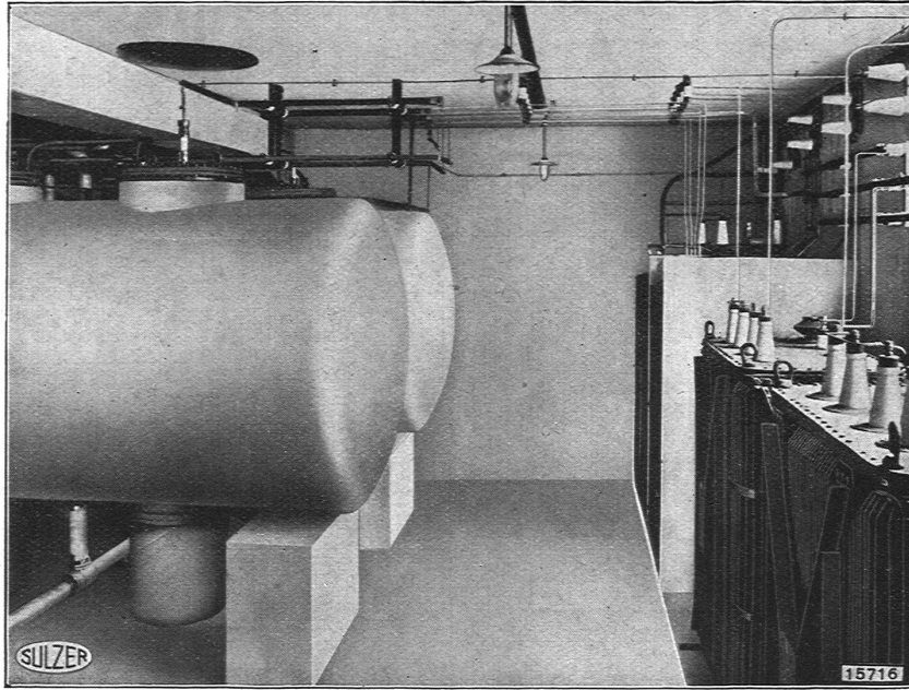
Elektro-Warmwasserspeicher von 1200 kW Einphasenwechselstrom, 1000 Volt, 16 \frac{2}{3} Per/sec. in der S.B.B.-Werkstätte Bellinzona.
