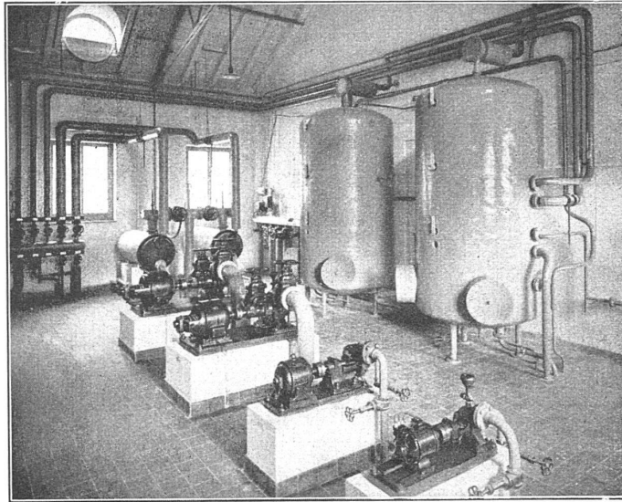
Zentrale einer Sulzer-Pumpenheizung und Warmwasserbereitung in einem Krankenhaus
