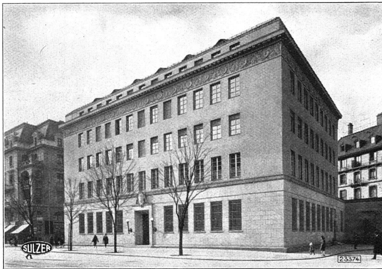
Schweiz. Nationalbank, Zweiganstalt Luzern. Sulzer-Pumpen-Warmwasserheizung, Warmwasserbereitung, Tresorheizungs- und Lüftungsanlage.
